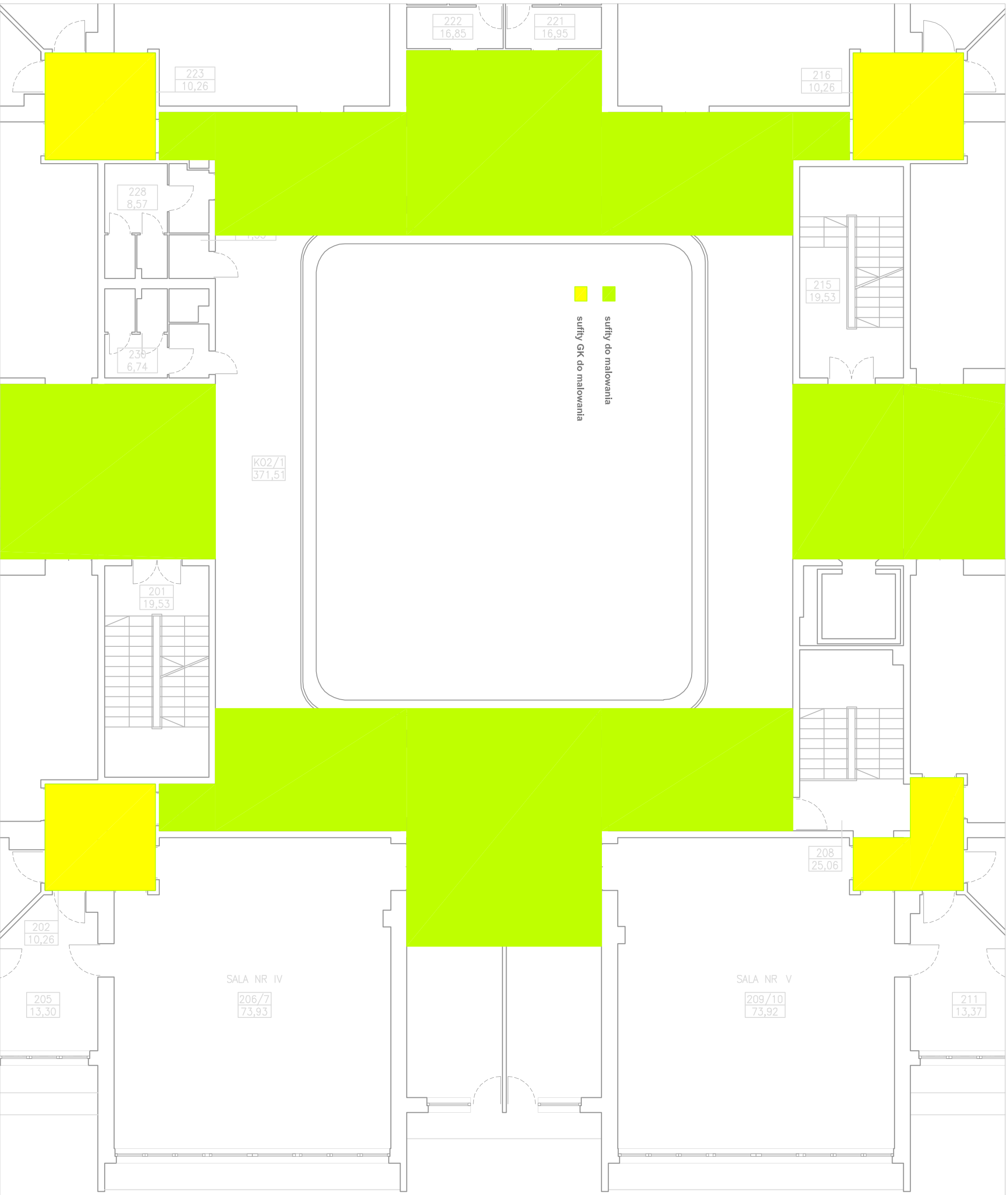
rys. 5 Projekt oświetlenia ogólnego komunikacji PIĘTRO 2 Plan sufitów do malowania Sąd rejonowy w Lubinie 59-300 Lubin ul. Wrocławska 3 skala 1:100 opracował:
